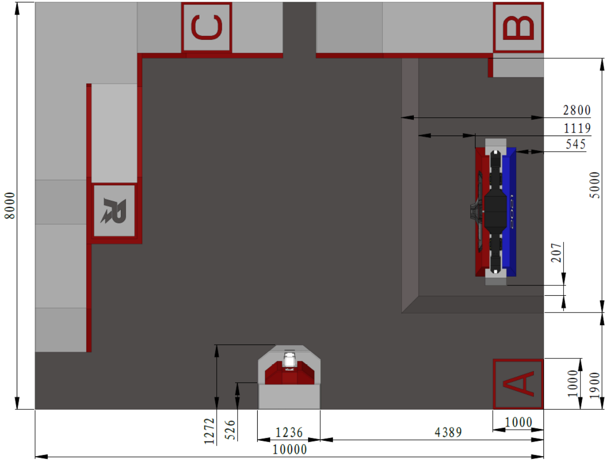
图 4-1 工程采矿场地示意图
