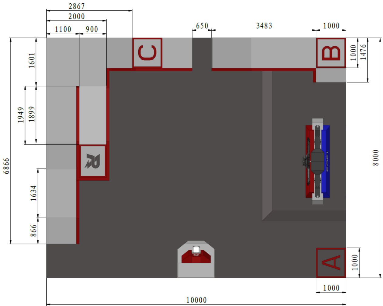
图 4-6 步兵竞速与智能射击场地模块示意图
