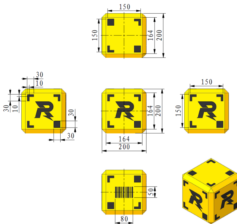
图 4-3 矿石示意图
