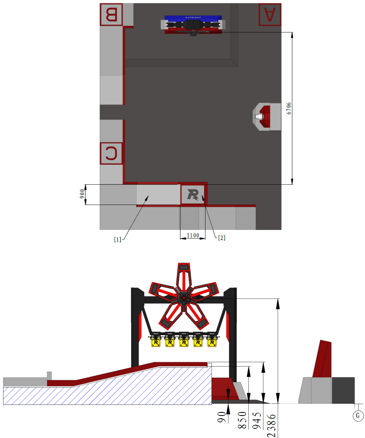
图 4-7 能量机关激活点尺寸示意图
