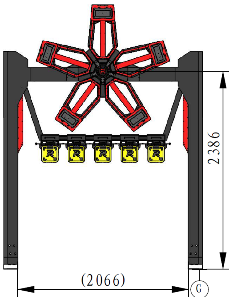
图 4-9 能量机关示意图
